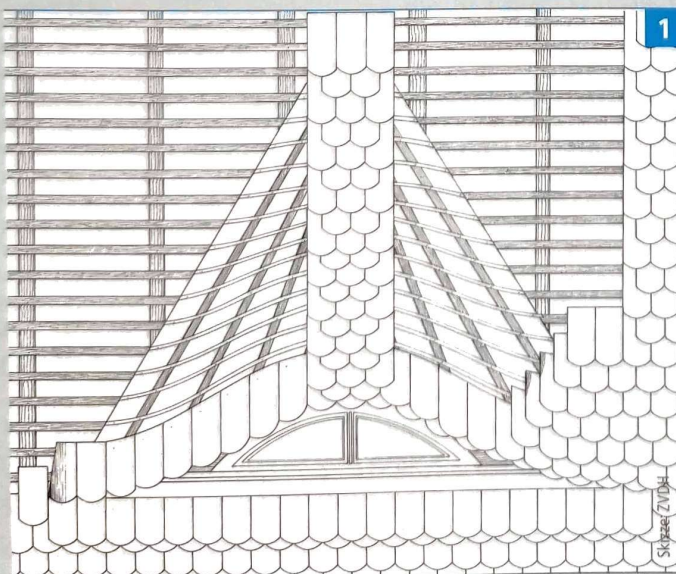
Eindeckung der Traufschichten an der Fledermausgaube
